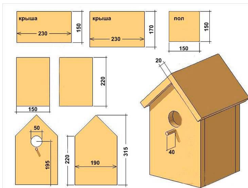
Чертеж 2. «Скворечник с двухскатной крышей»
